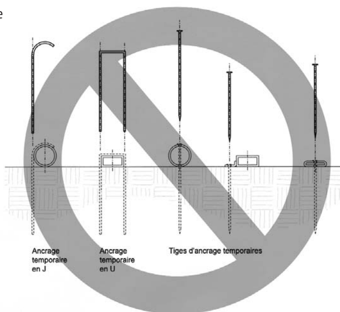
FIGURE 3 : Ancrages pour buts amovibles
