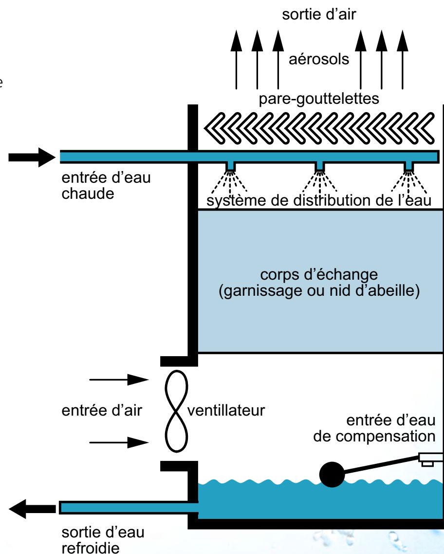
Figure 1 : Tour de refroidissement à l'eau
