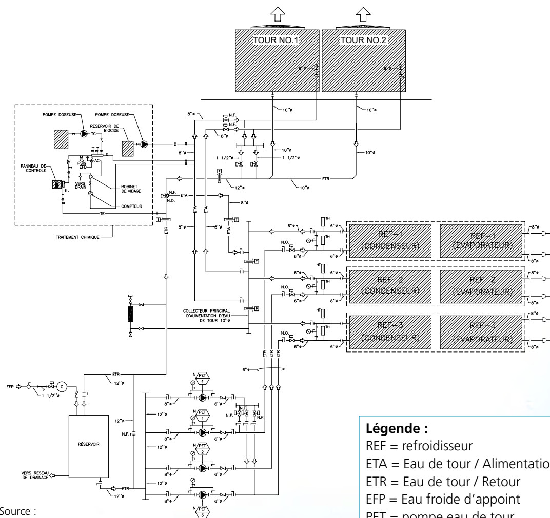
Figure 2 : Installation de tours de refroidissement à l'eau
