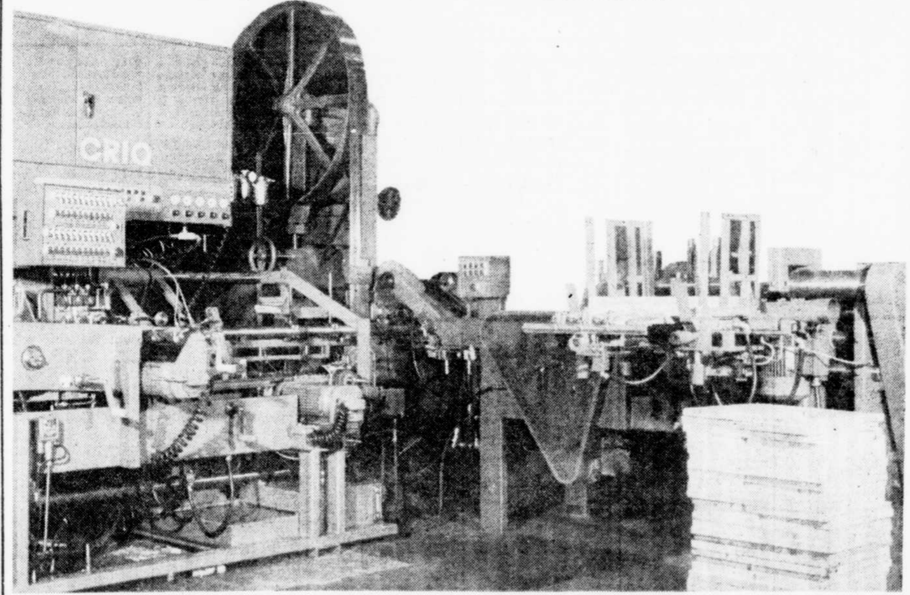
Cette machine, mise au point par le CRIQ pour fabriquer des côtés de tiroirs à partir de panneaux confectionnés de restes de bois collés et planés, fait le travail de sept machines. Un automate programmable contrôle le déroulement des opérations. Les côtés de tiroirs prêts à assembler sont fabriqués au rythme d'une paire toutes les dix secondes.
