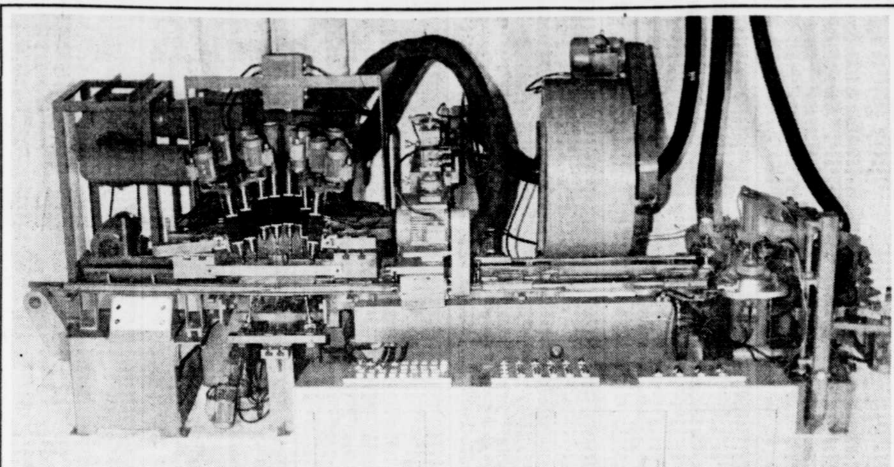
Une première mondiale dans l'industrie du meuble: une machine à fabriquer des fonds de chaises dont le concept revient au Centre de recherche industrielle du Québec.
