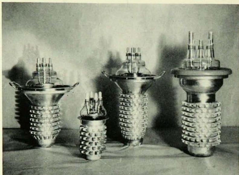
Les nouveaux tubes à filament de tungstène Thorié
