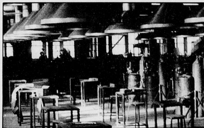
Hottes de captation au dessus des tables de soudure des étudiants dans un centre de formation.
