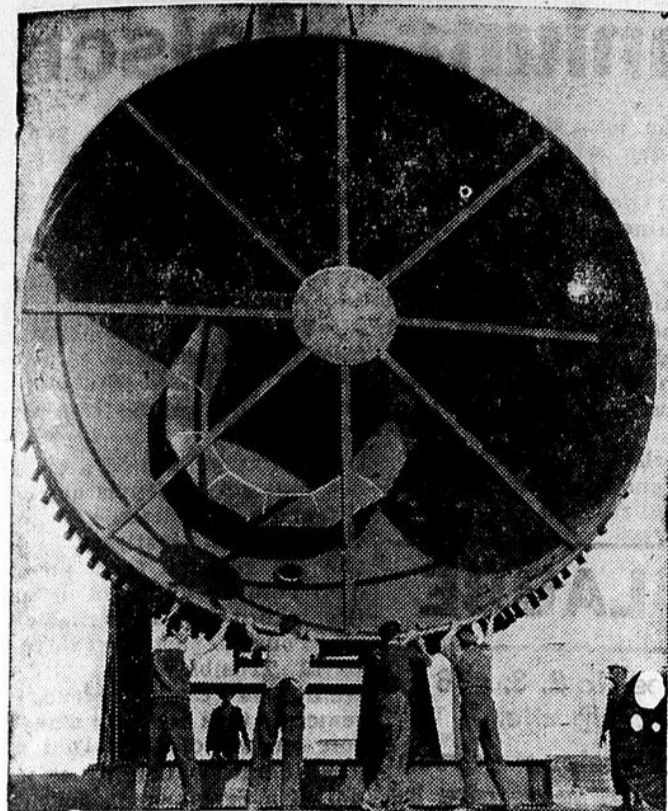
A Hinkley Point, Somerset, Angleterre, où ce qui est en construction probablement la plus grande station nucléaire au monde, voici une section en forme de dôme qui est placée en position pour être soudée à une série de sections d'anneaux de métal préfabriqués afin de former une cellule de production de vapeur pour diriger les turbo-alternateurs. Les coquilles de ces cellules ont 90 pds de hauteur et pèsent 390 tonnes. Il y aura six cellules à chacun des deux réacteurs.
