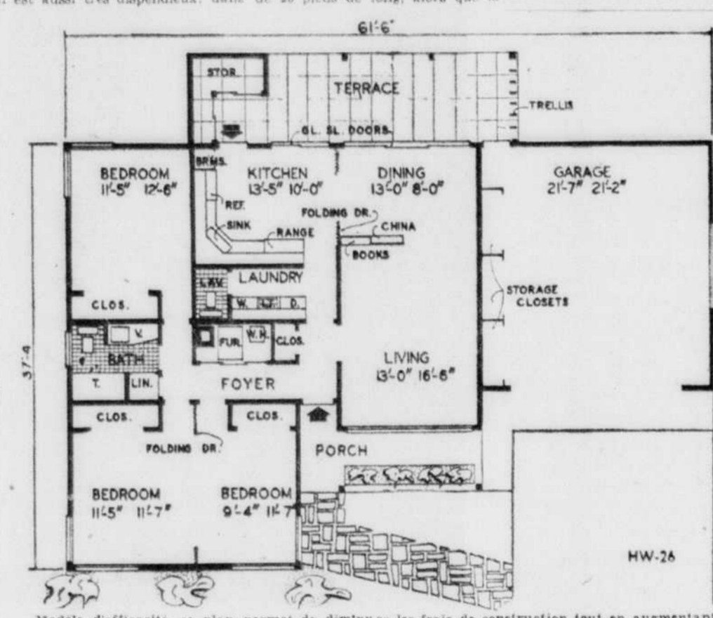
Modèle d'efficacité, ce plan permet de diminuer les frais de construction tout en augmentant le nombre de ses commodités.
