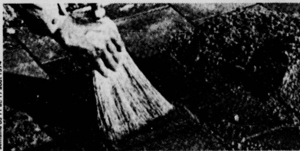
FIGURE 4: Après avoir posé tous les blocs, passez légèrement le balai entre chacun des blocs afin d'éliminer le surplus de sable. Puis, vous arrosez la surface couverte à l'aide d'un boyau, afin que le sable prenne une position ferme entre chacun des blocs. N'arrosez toutefois que la surface dure pour éviter de creuser davantage l'espace requis entre les blocs. Vous pourrez évidemment vous faciliter la tâche en utilisant le catalogue illustré DECO-PLANS qui vous offre plusieurs idées originales pour votre patio comme pour le reste de votre maison. Vous n'avez qu'à utiliser le coupon qui apparaît dans les pages de cette chronique. Bonne chance.
