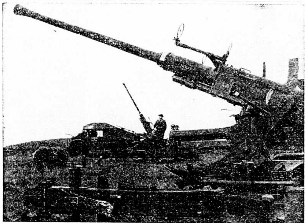
SUR LES COTES DU PACIFIQUE. — Ces canons antiavions Bofors de fabrication canadienne, remorqués par des tracteurs canadiens, protègent nos côtes sur le nouveau front du Pacifique. Ces pièces ont un pouvoir-feu de 140 obus à la minute.
