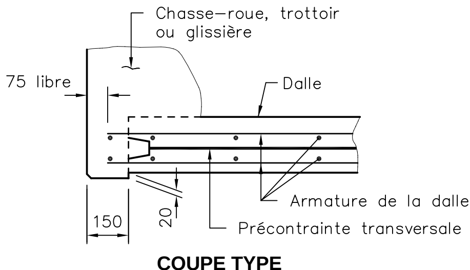
Figure 8.3.3 Précontrainte transversale
