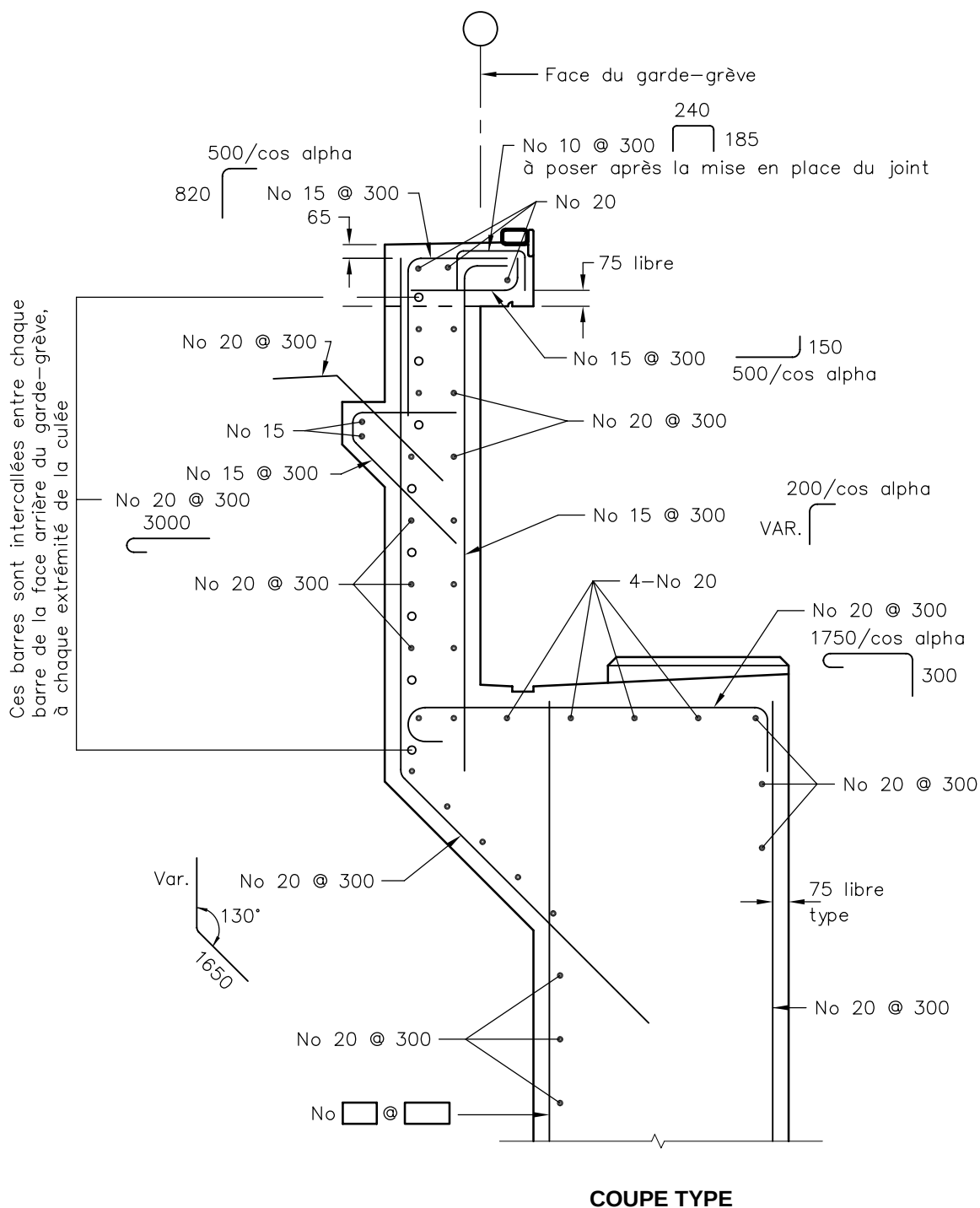
Figure 11.3-6 Culée-galerie avec joint de tablier (armature)
