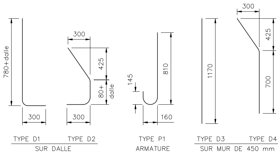
Figure 12.2-7 Glissière en béton type 202
