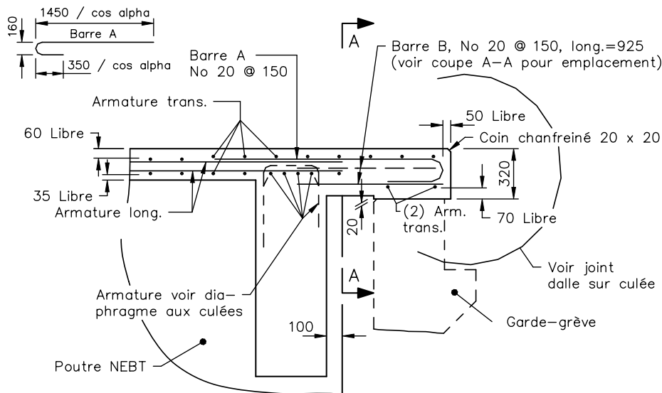
PROFIL - POUTRE PRÉFABRIQUÉE EN BÉTON PRÉCONTRAIT
