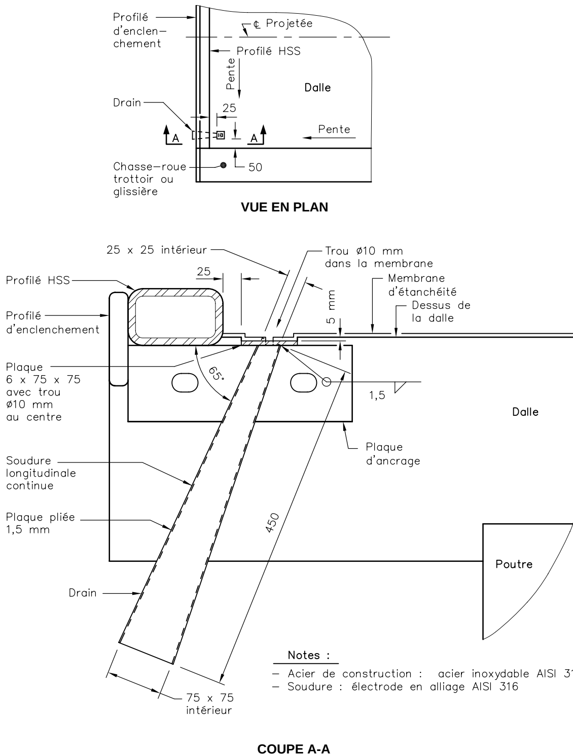
Figure 2.2-2 Drain d'interface
