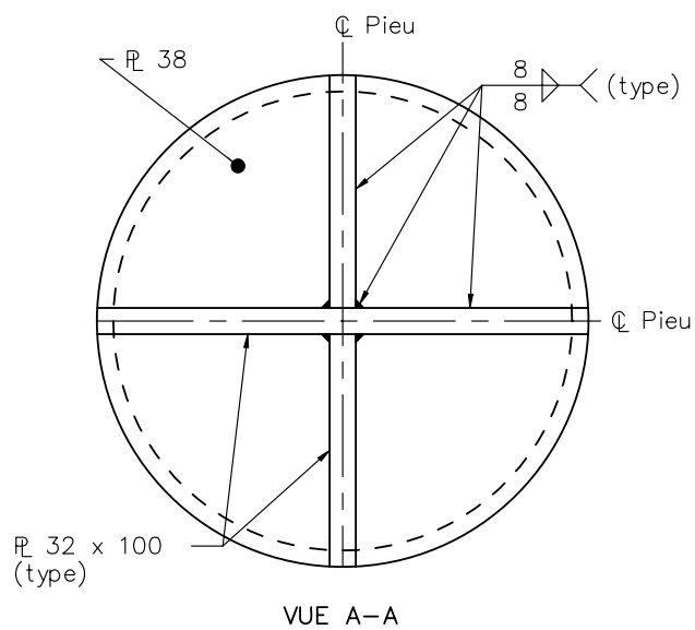
Figure 6.5-2 Pointe conventionnelle pour pieu tubulaire en acier
