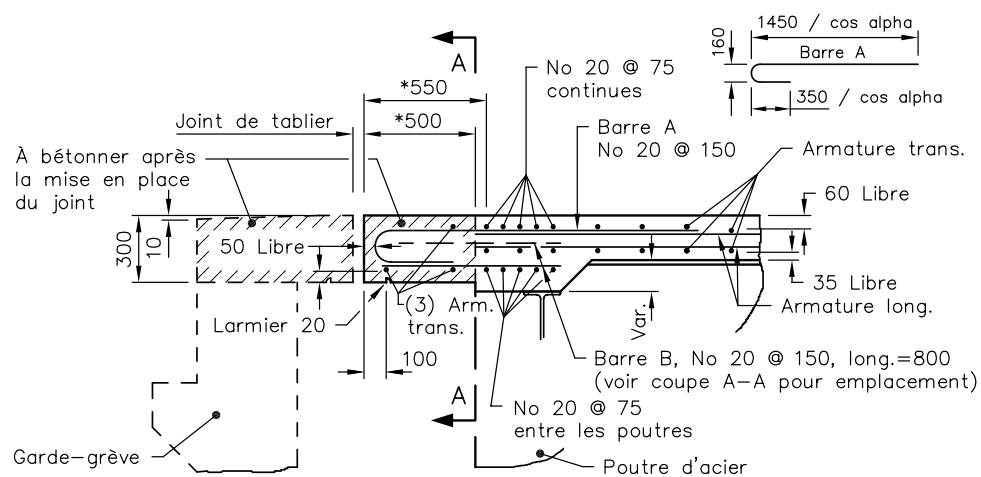
PROFIL - POUTRE EN ACIER
