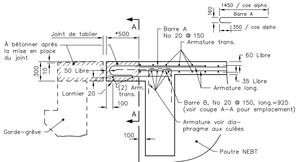
PROFIL - POUTRE PRÉFABRIQUÉE EN BÉTON PRÉCONTRAIT
