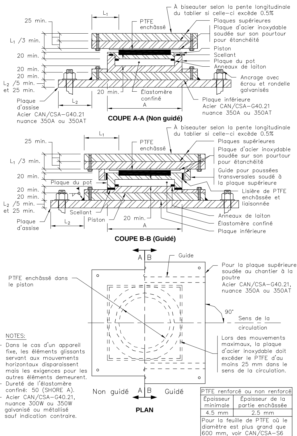
Figure 11.2-3 Appareil d'appui à élastomère confiné remplaçable
