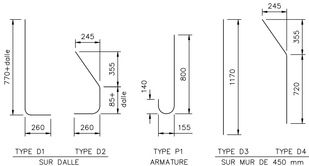
Figure 12.2-6 Glissière en béton type 201
