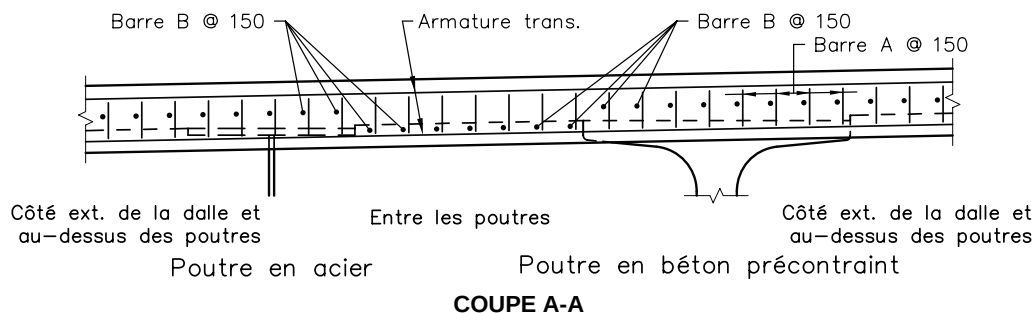
COUPE A-A
