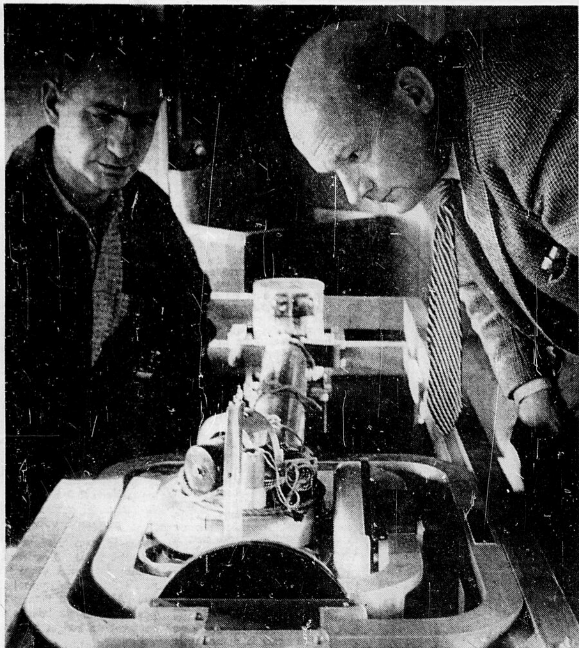
Weldon Hannaford, agent responsable, et Paul Serson, chef de la Division du géomagnétisme (à droite) vérifient le magnétomètre aéroporté à trois composantes.
