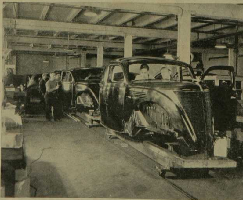
ON CONSTRUIT MAINTENANT, AUX USINES DE LA FORD MOTOR COMPANY OF CANADA, À WINDSOR, EN ONTARIO, LA NOUVELLE VOITURE FORD-LINCOLN, LA LINCOLN-ZÉPHYR À DOUZE CYLINDRES EN V. DANS LA VIGNETTE DU HAUT, M. WALLACE R. CAMPBELL, PRÉSIDENT DE LA FORD MOTOR OF CANADA, EXAMINE LA PREMIÈRE VOITURE DE CETTE MARQUE ASSEMBLÉE AU CANADA. VIGNETTE DU BAS : L'AUTO DANS LA DERNIÈRE PHASE DE L'ASSEMBLAGE.
