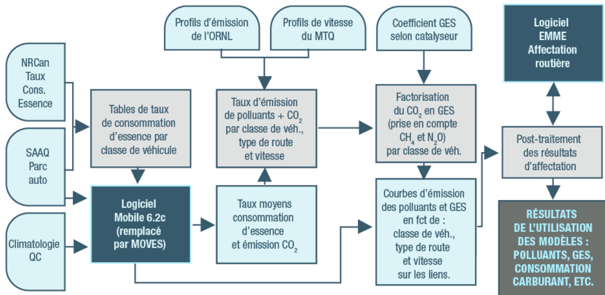
Figure 4. Schéma simplifié de l'utilisation des modèles de circulation routière
