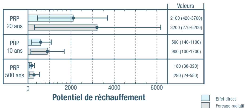
Figure 7. Potentiel de réchauffement planétaire du carbone noir sur des périodes de 20, 100 et 500 ans
