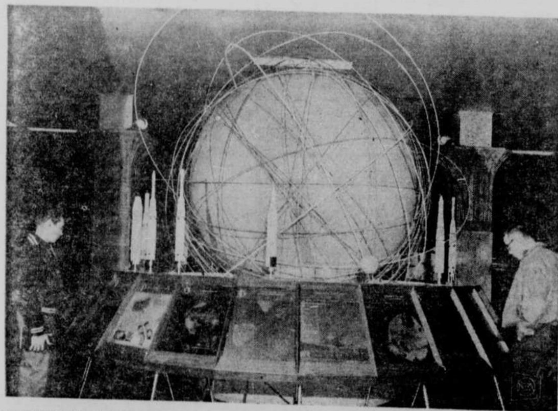
LA TERRE BIEN ENCERCLEE. — Cette sphère terrestre apparaît ici comme une énorme balle dont les fils ont été démelés. On peut l'examiner dans un exhibit consacré à l'ère spatiale que présente à Cleveland un institut de technologie. On y découvre chacun des trajets suivis par presque tous les satellites récents lancés par les Etats-Unis et la Russie. Cet exhibit, assure-t-on, qui a coûté plus de $50,000, est unique en son genre.
