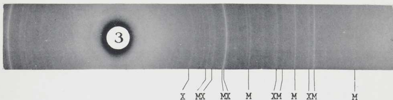
PLANCHE IV — Diagramme de diffraction des rayons X* des substances trouvées dans les échantillons de matte et de scorie:
