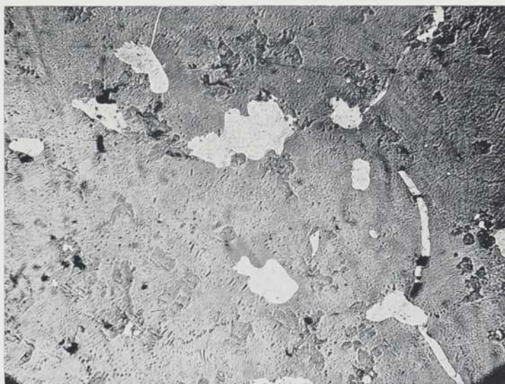
PLANCHE II A — 53.2 p. 100 de matte de cuivre —x100 Bornite avec taches de cuivre métallique.
