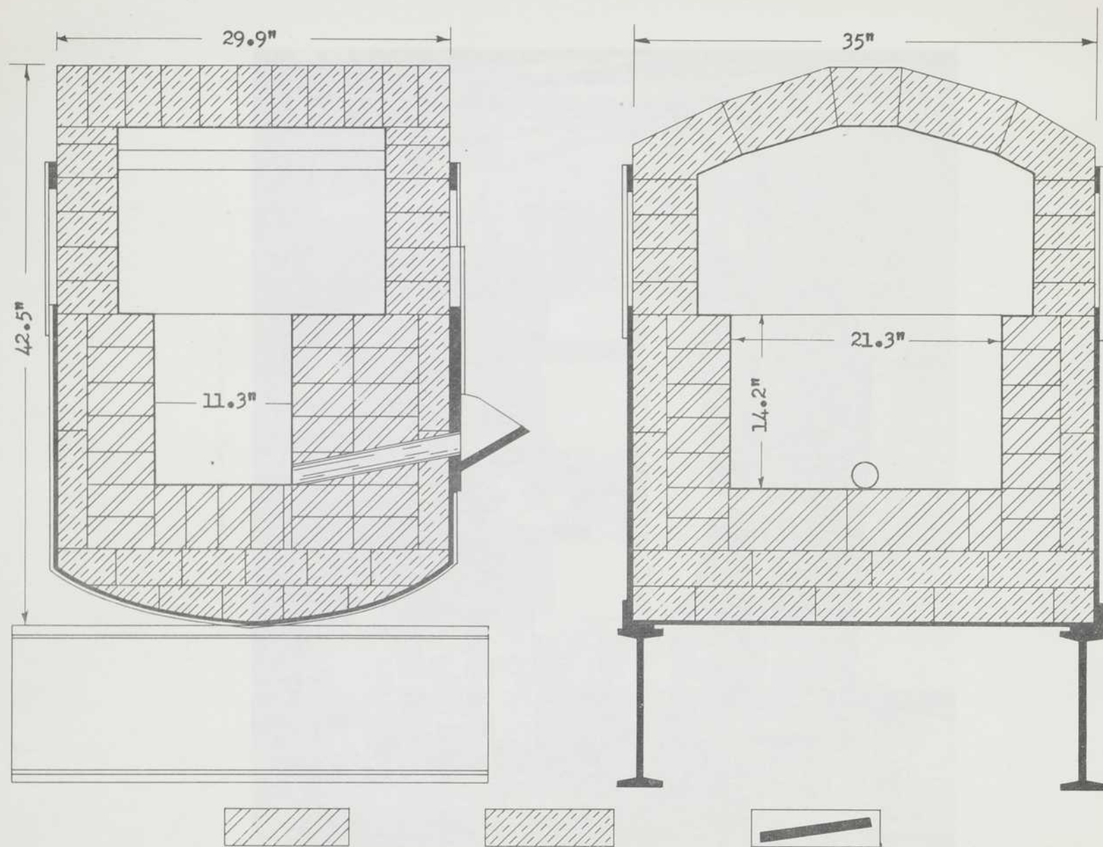
Figure V. Section centrale de four expérimental, avec dimensions.
