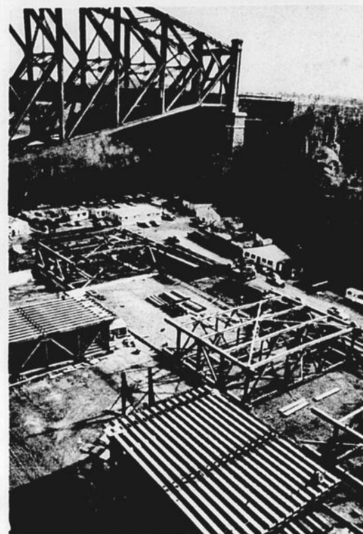
A gauche, sous le pont de Québec, on aperçoit à marée basse, au premier plan, les débris de la section tombée autrefois dans le fleuve; ci-dessus, le chantier de la rive sud où on assemble les sections du tablier.
