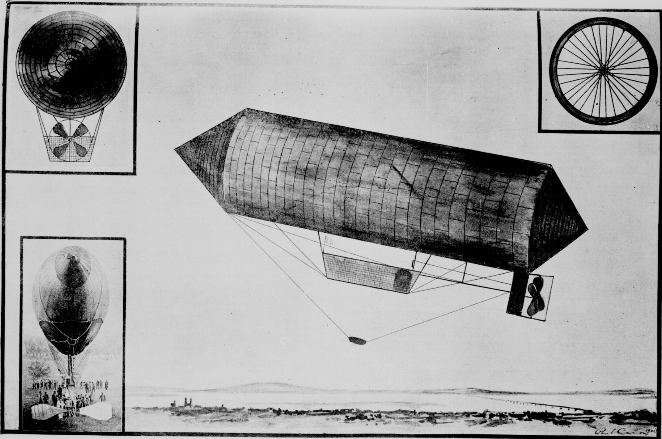
Dessin du ballon que M. Louis Fillion, de Montréal, est en voie de construire pour disputer à Santos-Dumont la solution du problème des ballons dirigeables. A gauche, dans le coin supérieur, une coupe transversale du ballon, indiquant la position particulière de l'hélice. A droite, illustration du principe de la charpente. A gauche, dans le bas, le type ordinaire des ballons dirigeables d'aujourd'hui. (Pour plus amples détails, voir page 194)
