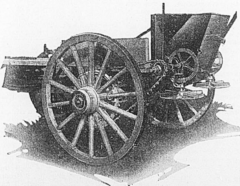
La Monsarrat Machinery & Foundries Limited vient de mettre sur le marché un nouvel épandeur de chaux et d'engrais chimique que l'on prétend particulièrement pratique lorsque l'engrais chimique a absorbé un peu d'humidité. Il peut même servir à semer de la graine.
