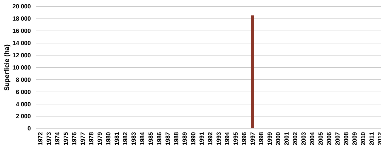
Figure 6 Superficie annuelle brûlée (ha) dans l'UA 085-62 entre 1972 et 2012 5,6
