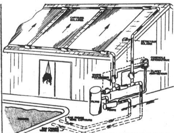
Dessin schématique d'un chauffe-piscine solaire.
