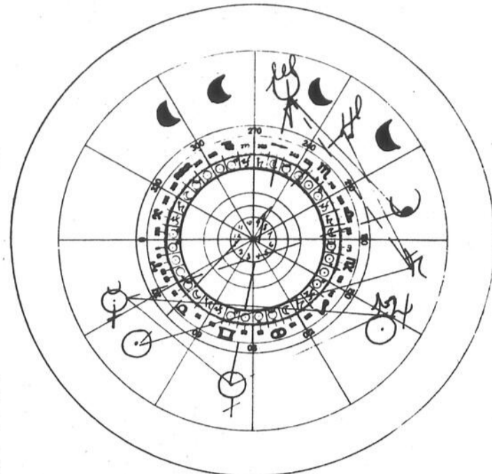
Le ciel de la semaine du 30 avril au 7 mai 1980. Telle sera la position de chaque planète.
