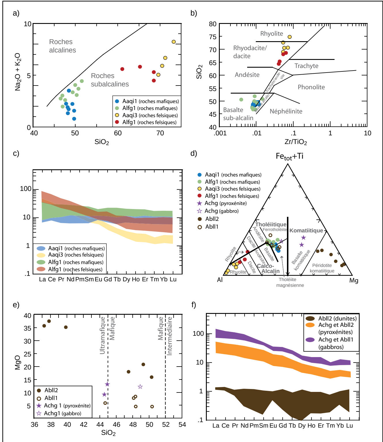
FIGURE 5 - Diagrammes géochimiques des roches volcaniques et des intrusions mafiques et ultramafiques de la région du réservoir Laforge 1 : a) diagramme discriminant binaire de Irvine et Baragar (1971); b) diagramme de classification binaire de Winchester et Floyd (1977); c) diagramme des ÉTR normalisés aux chondrites de Sun et McDonough (1989) pour les roches volcaniques; d) diagramme discriminant ternaire de Jensen (1976); e) diagramme binaire MgO versus SiO 2 ; f) diagramme des ÉTR normalisés aux chondrites de Sun et McDonough (1989) pour les intrusions ultramafiques.
