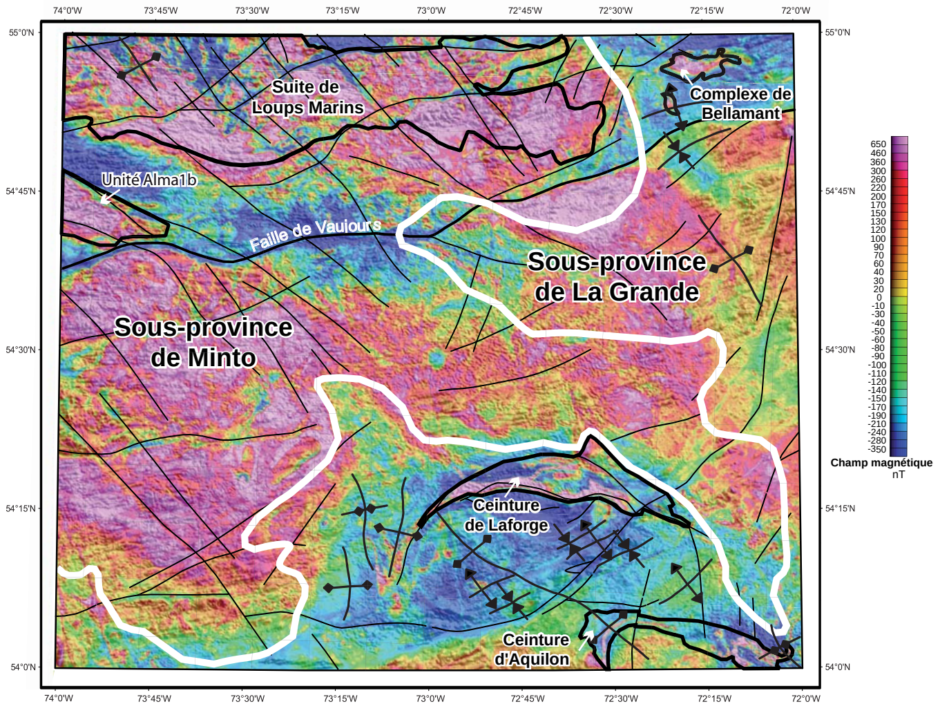
FIGURE 4 - Composante résiduelle du champ magnétique total avec relief topographique ombragé de la région de Laforge 1 (modifiée de Goldak Airborne Surveys, 2008).
