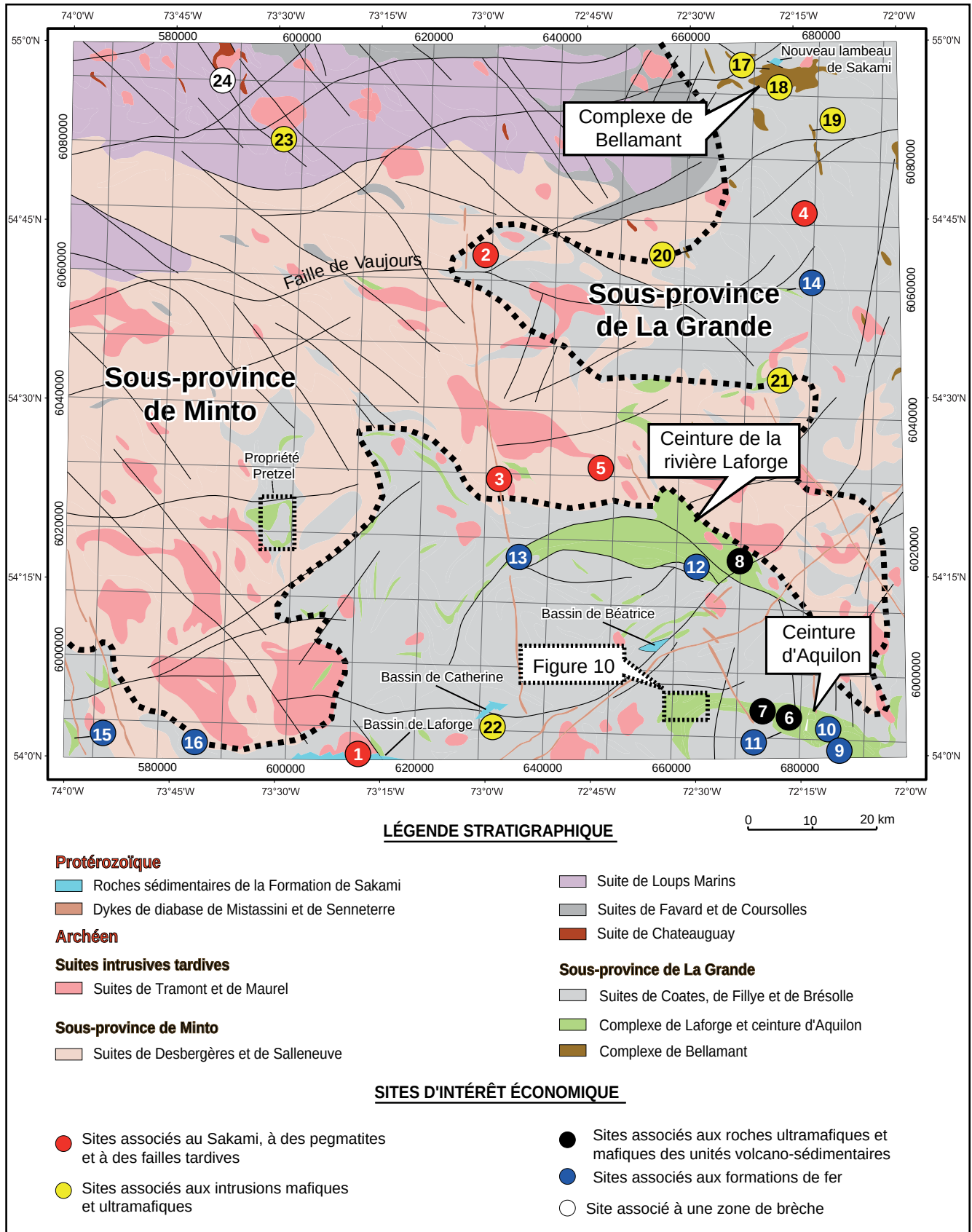
FIGURE 9 - Localisation des principaux sites d'intérêts économiques de la région du réservoir Laforge 1. Les numéros font référence aux sites décrits dans le tableau 4.
