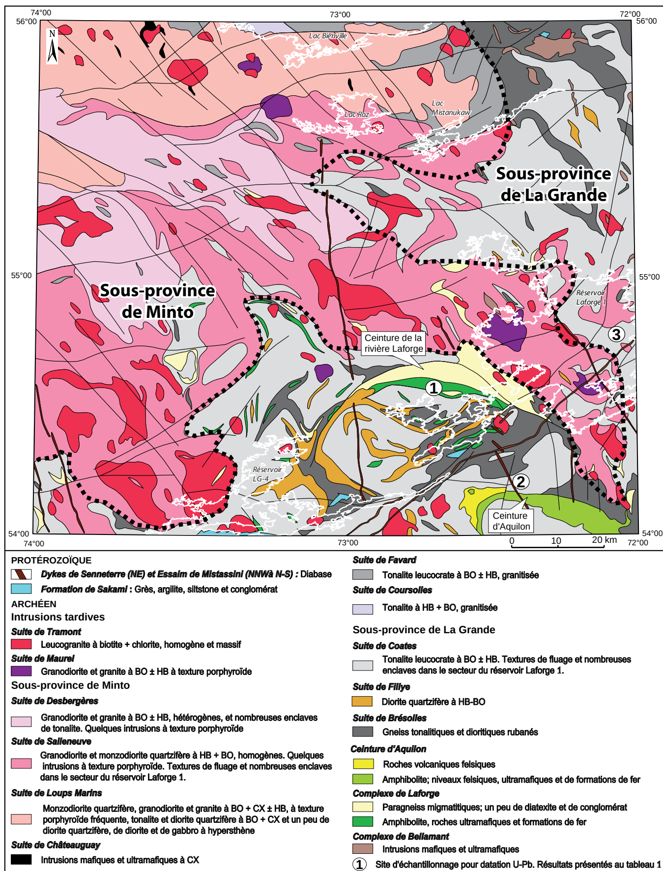
FIGURE 3 - Géologie simplifiée de la région du réservoir Laforge 1.
