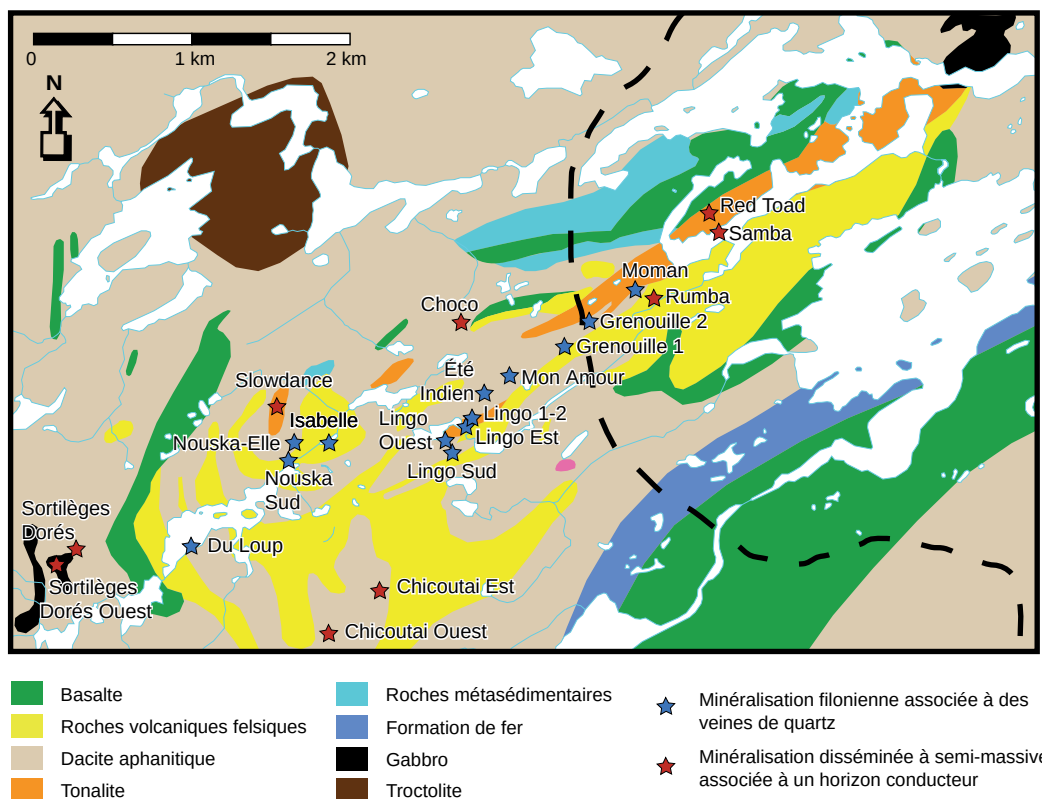
FIGURE 10 - Géologie simplifiée et localisation des principaux indices et de la partie ouest de la Ceinture d'Aquilon (modifiée de Moar, 2007b).
