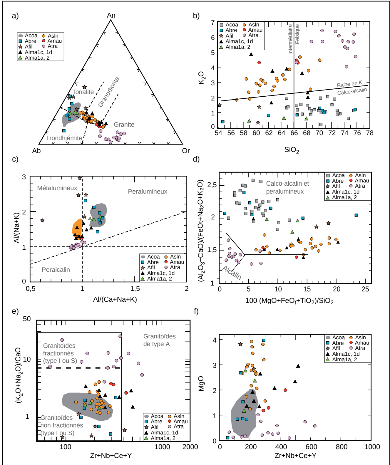
FIGURE 6 - Diagrammes géochimiques des roches intrusives felsiques et intermédiaires de la région du réservoir Laforge 1 : a) diagramme de classification normative albite-anorthite-orthose de O'Connor (1965); b) diagramme binaire K 2 O versus SiO 2 ; c) diagramme de l'indice de saturation en alumine de Maniar et Piccoli (1989); d) diagramme discriminant de Sylvester (1989); e) diagramme discriminant de Whalen et al. (1987); f) diagramme binaire MgO versus Zr+Nb+Ce+Y.
