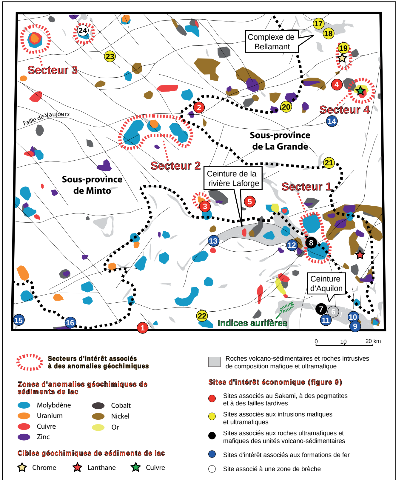
FIGURE 11 - Anomalies et cibles géochimiques de sédiments de lac déterminées par Lamothe (2009 et 2010) et correspondance avec les sites d'intérêts de la figure 9.
