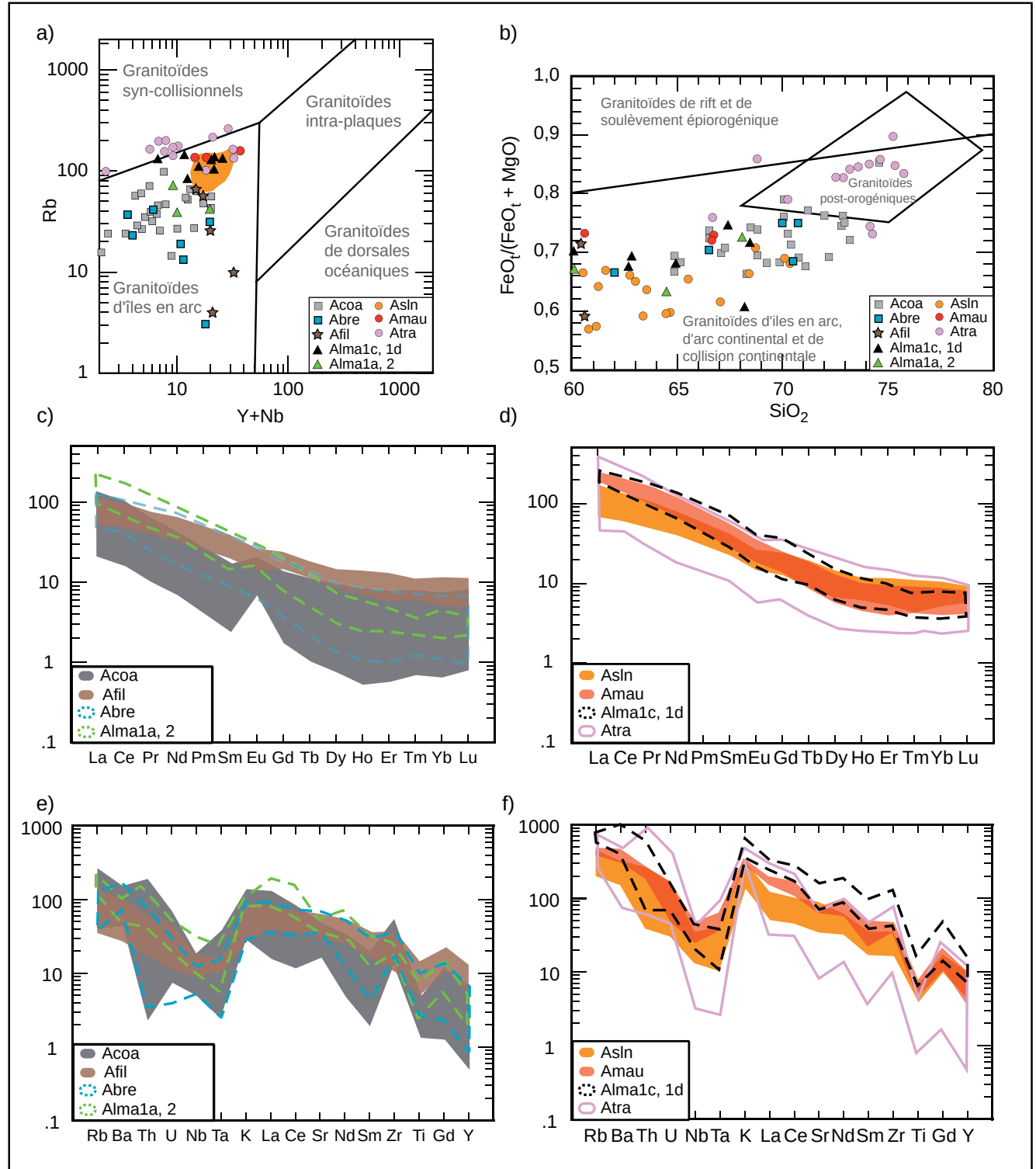
FIGURE 7 - Diagrammes géochimiques des roches intrusives felsiques et intermédiaires de la région du réservoir Laforge 1 : a) diagramme discriminant de Batchelor et Bowden (1985); b) diagramme discriminant de Maniar et Piccoli (1989); c) diagramme des ÉTR normalisés aux chondrites de Sun et McDonough (1989) pour les roches de composition tonalitique et dioritique; d) diagramme des ÉTR normalisés aux chondrites de Sun et McDonough (1989) pour les roches intrusives potassiques; e) diagramme des multiéléments normalisés aux chondrites de Sun (1980) pour les roches de composition tonalitique et dioritique; f) diagramme des multiéléments normalisés aux chondrites de Sun (1980) pour les roches intrusives potassiques.
