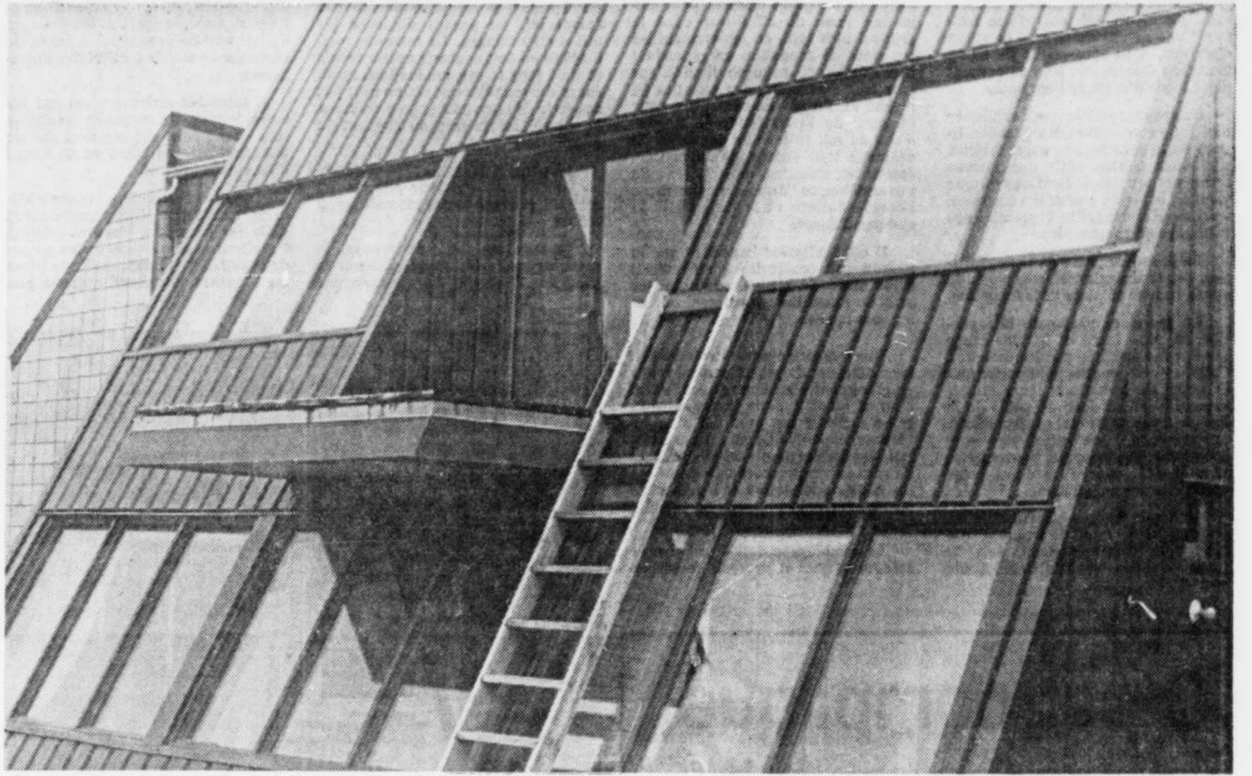
Un système simple pour bénéficier de l'énergie solaire: l'orientation et l'inclinaison des fenêtres du côté sud de la maison.
