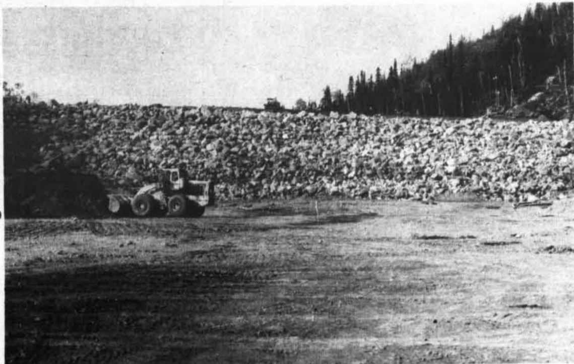
Le réservoir de régularisation de la rivière aux Outardes sera créé par huit barrages dont voici le premier terminé, le barrage no 6. Long de 500 pieds et haut de 90 pieds, ce barrage a un volume de 280000 verges cubes. Les deux principaux barrages auront un volume, le premier de 10 millions de verges cubes et, le second, de 6 millions. Sauf modification du programme, la mise en eau du réservoir débutera le printemps prochain. Les centrales Outardes 4 (632000 kilowatts) et Outardes 3 (745000 kilowatts) seront mises en service en 1969, tandis que la centrale Outardes 2 (454000 kilowatts) suivra en 1971.
