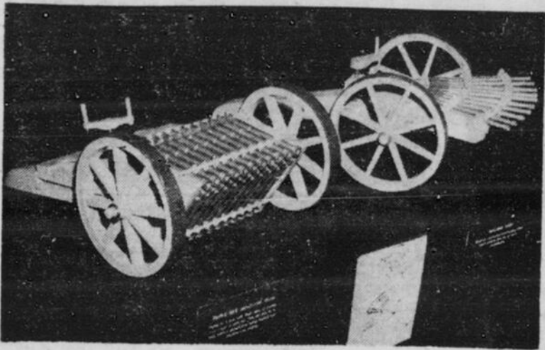
L'EXPOSITION DE VINCI A MONTREAL. — Notre photo montre, ci-haut, une invention de Léonard de Vinci que son époque dut considérer pour le moins révolutionnaire. Il s'agit d'un genre de canon-mitrailleur de 33 tubes divisés en trois groupes. Tandis qu'une rangée pointe vers l'ennemi l'autre rangée se refroidit. Pendant ce temps on recharge la dernière. Cette pièce, à échelle, fait partie de la collection du Dr Roberto Guatelli, exposée présentement aux bureaux de l'International Business Machines, à Montréal, jusqu'au 23 octobre prochain.
