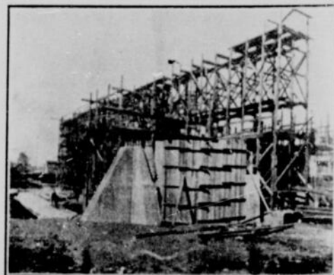
Autre vue de l'échafaudage établi pour la construction de l'élevateur
