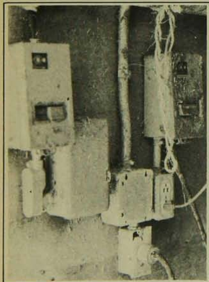
Des boîtes de contrôle sales et humides sont des causes de mal fonctionnement des moteurs et, parfois, d'incendie ou d'électrocution.
