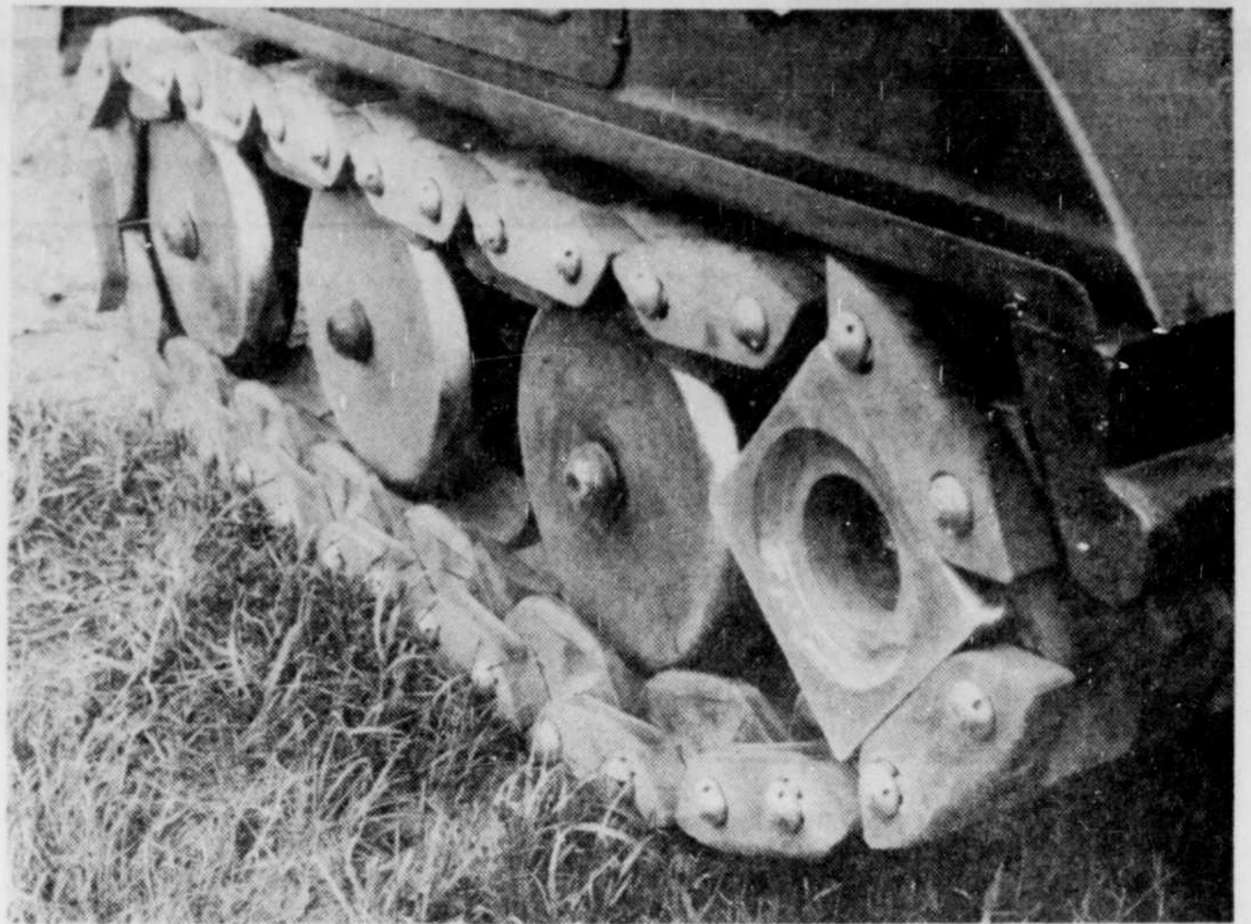
CETTE CHENILLE DE CAOUTCHOUC, fabriquée par Martin Manufacturing du Cap-de-la-Madeleine, est une découverte révolutionnaire reconnue par Muskeg Research
