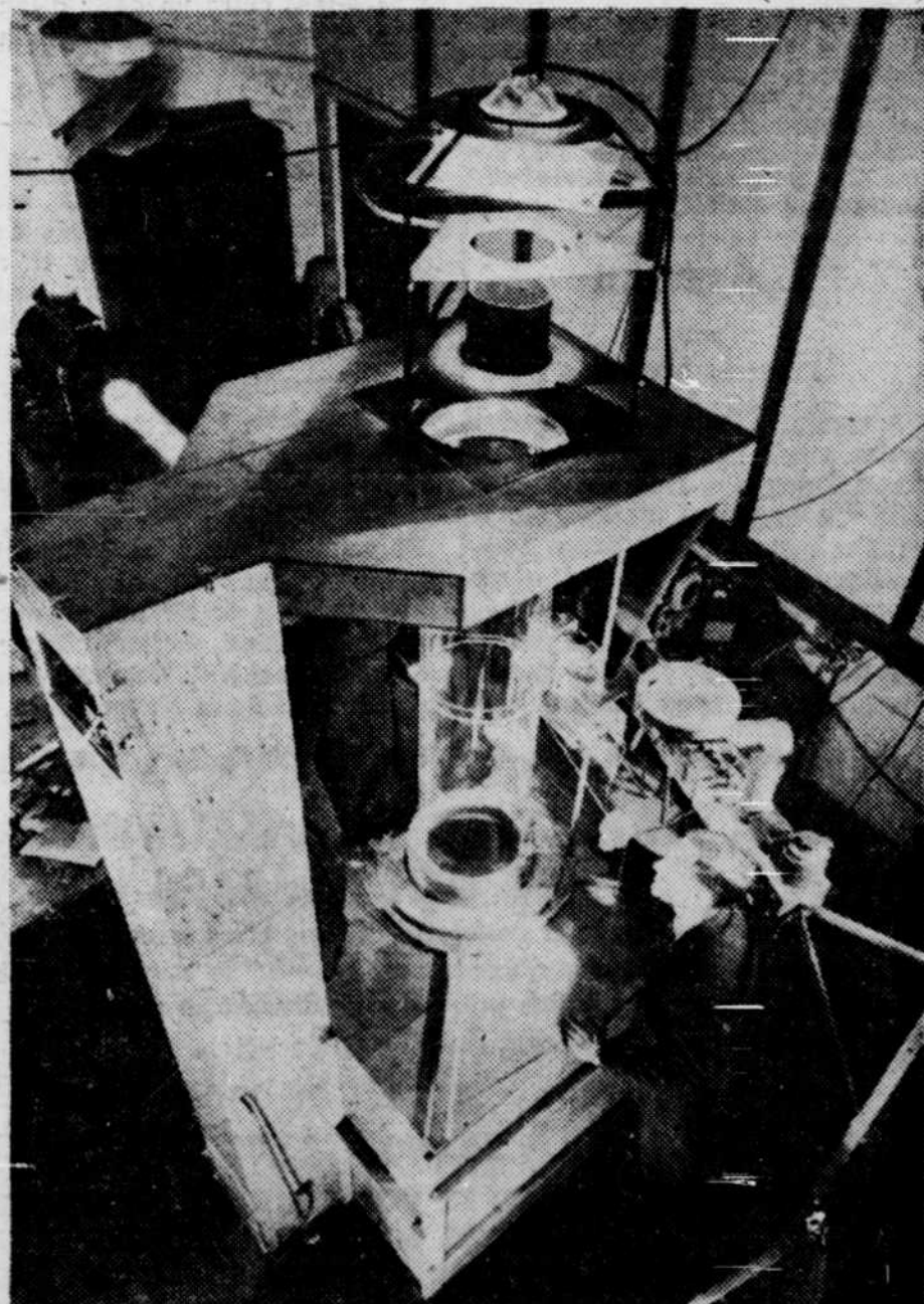
La "chambre à nuages" mise au point par la CSIRO pour recréer artificiellement les conditions qui règnent dans un "nuage non-glacé". Cet appareil est un cylindre de verre d'environ 3,50 mètres de haut, où l'on fait passer de l'air et dans lequel on vaporise de l'eau par une fente pratiquée dans la paroi. Grâce à la "chambre à nuages", les savants australiens ont pu suivre le processus de la "pluie non glacée": ils ont vu les gouttelettes d'eau emportées vers le haut par le courant d'air, entrer en collision, puis tomber. On a d'ailleurs enregistré ce processus sur film pour permettre une étude plus détaillée.
