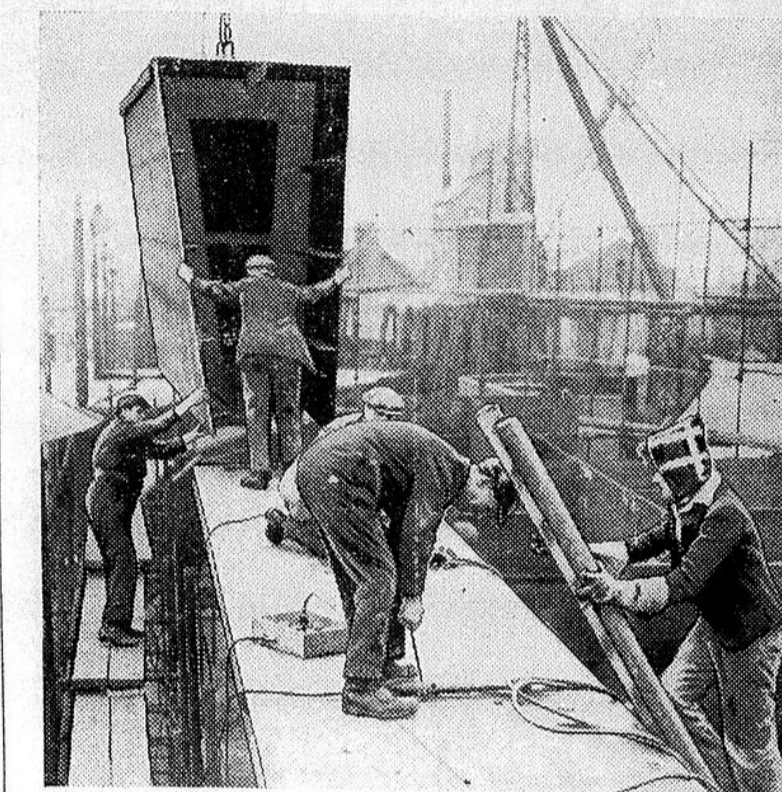
Des ouvriers des chantiers maritimes Henry Scarr, à Hull, en Angleterre, assemblent les parties d'un navire.
