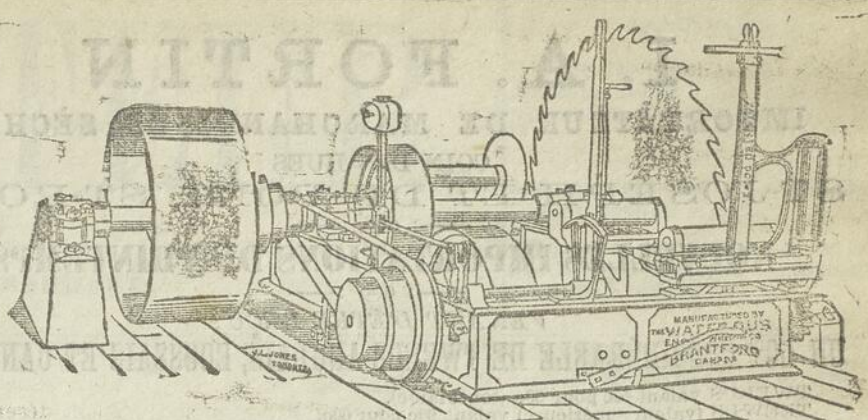
Moulins à Seie. —Sept grandeurs avec toutes les dernières améliorations. Echantillons à voir au magasin.
