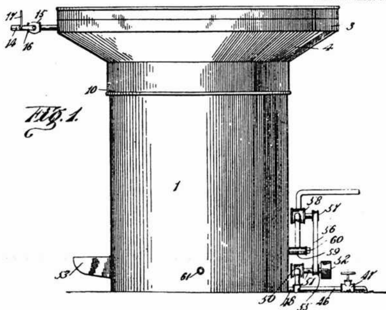
Vue Extérieure
