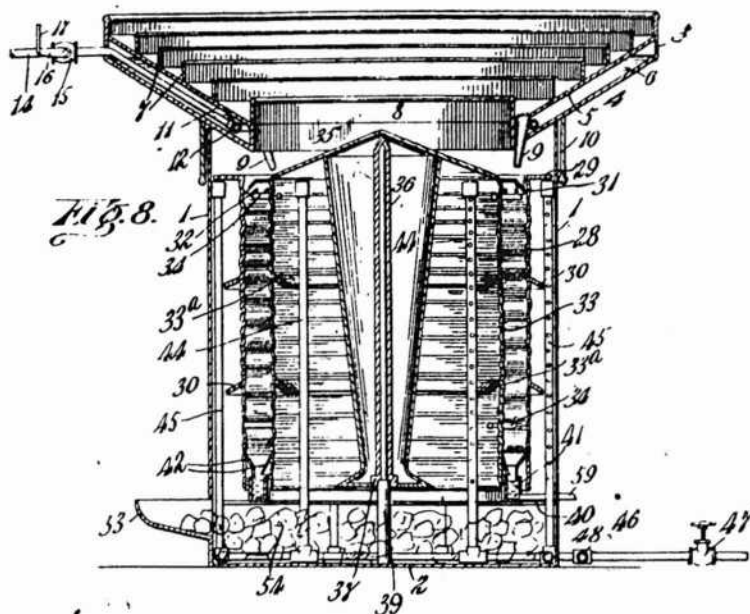
Vue Intérieure
