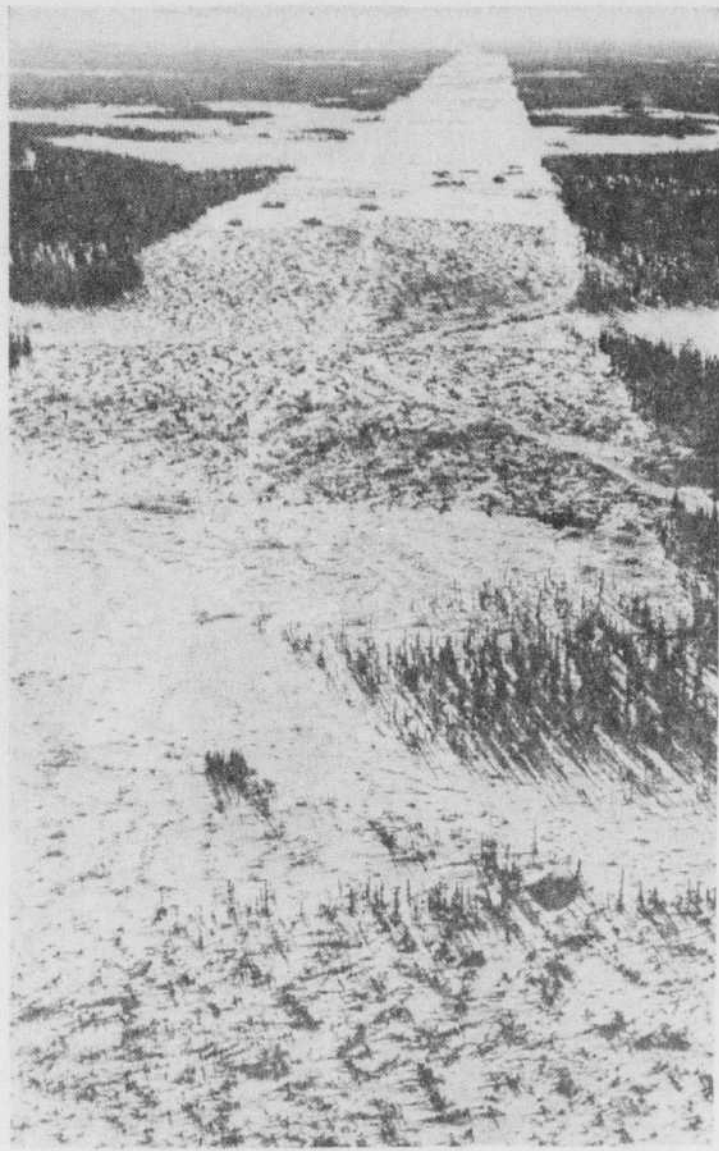
LE PASSAGE DES LIGNES — Cette vue aérienne d'un passage large de 710 pieds indique la voie que prendront les trois lignes de transmission de 735.000 volts chacune, pour transporter l'électricité qui sera produite par l'usine hydroélectrique des chutes Churchill, dans le Labrador central. On prévoit commencer la livraison de l'énergie le 1er mai 1972, et parachever en 1976 les travaux de $950 millions.
