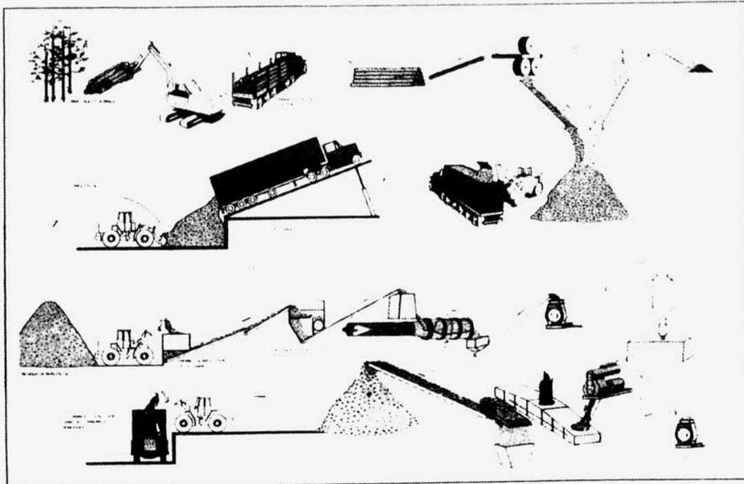
Le présent schéma montre à quel point l'intervention humaine est limitée dans l'ensemble du processus de production des granules "Woodex".
