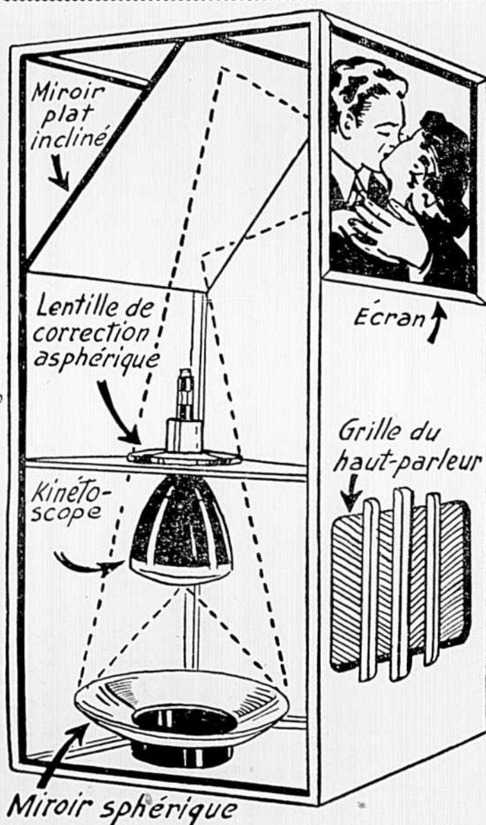
Ce nouveau modèle d'appareil récepteur de télévision privé assure la projection sur un écran de plastique faisant partie de l'appareil. On trouvera ci-contre l'explication du fonctionnement de cet appareil récepteur.
