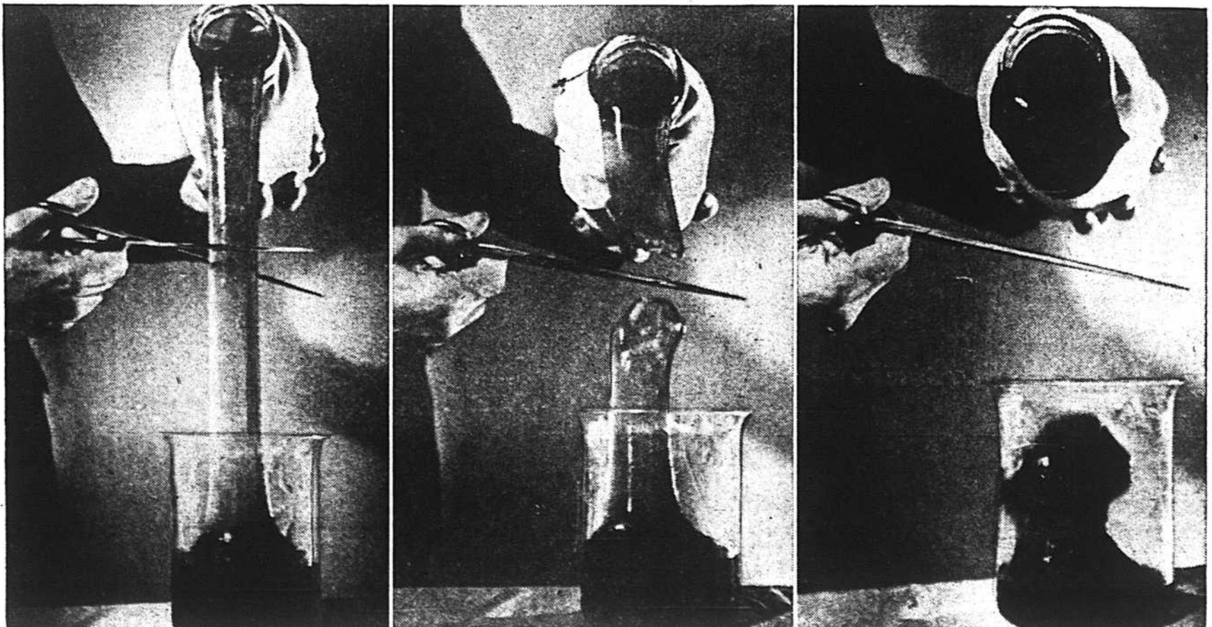
Le comportement élastique d'un fluide peut être assez étonnant, mais il pose aussi des problèmes. Dans les photos ci-dessus, on fait couler un fluide, on le coupe pendant l'écoulement, et la partie supérieure se rétracte jusqu'au bocal.
