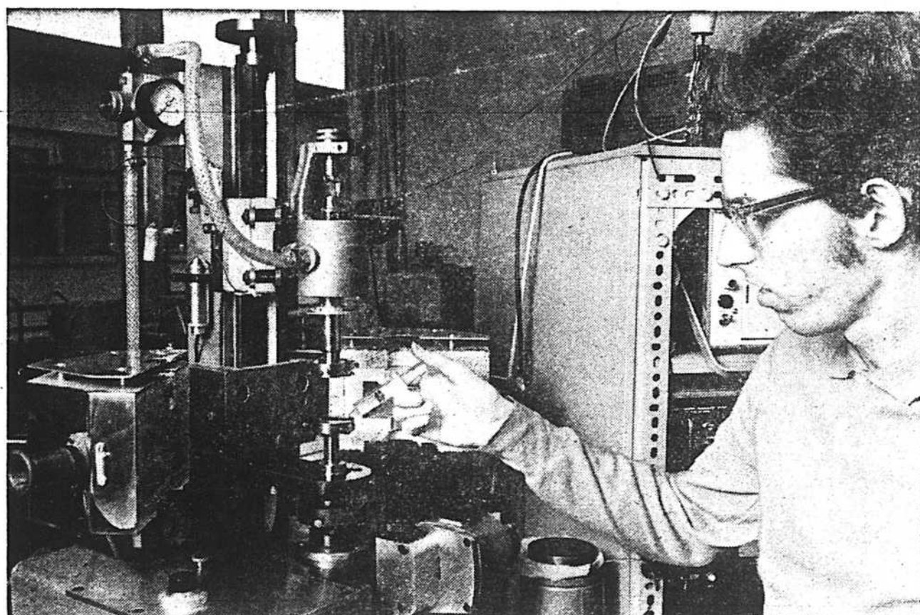
Le rhéogoniomètre de Weissenberg, un appareil de précision, qui permet d'étudier les propriétés particulières des non-Newtoniens, comme l'élasticité, la viscosité et les efforts normaux.
