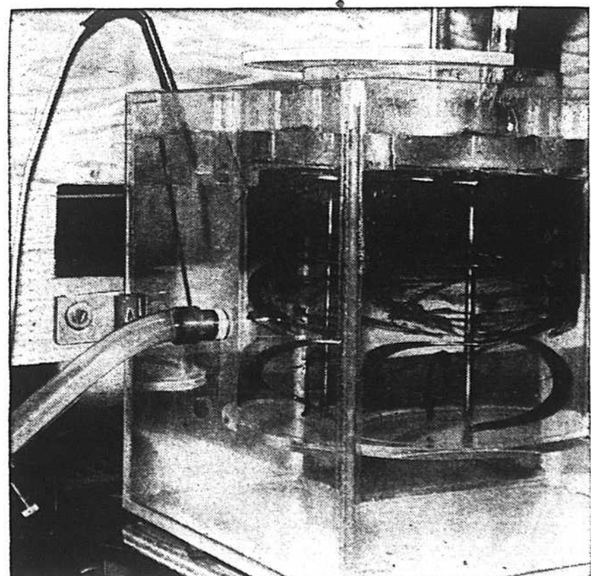
Les non-Newtoniens ont une réaction particulière au malaxage. Cet agitateur hélicoïdal indique justement au spécialiste que les mélanges s'exercent le long de la paroi de l'agitateur.
