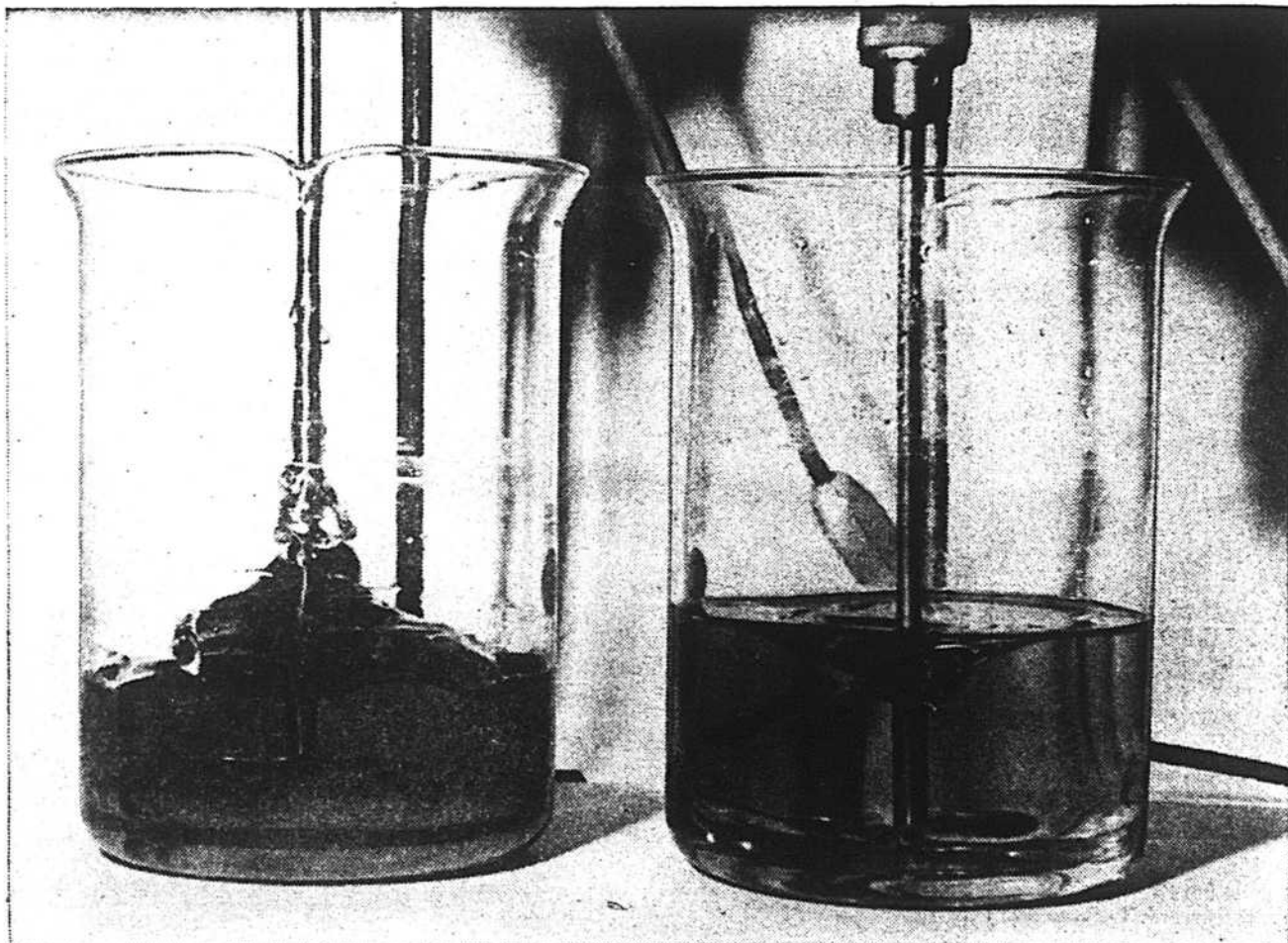
A gauche, un non-Newtonien, avec vortex inversé. Ce qui veut dire, en somme, que ce fluide a des propriétés élastiques, et qu'il a tendance à monter le long de l'agitateur, plutôt que de réagir comme le fluide Newtonien de droite, pourtant visqueux, qui a tendance à s'éloigner du centre de l'agitateur.
