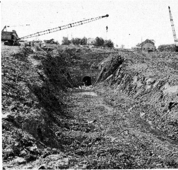
Canal d'entrée du futur lit de la Yamaska près du nouveau barrage en construction à Savage Mills, à l'est de Granby.
