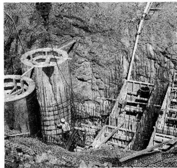
Le complexe des régulateurs du niveau des eaux en construction près du futur barrage de Savage Mills.
