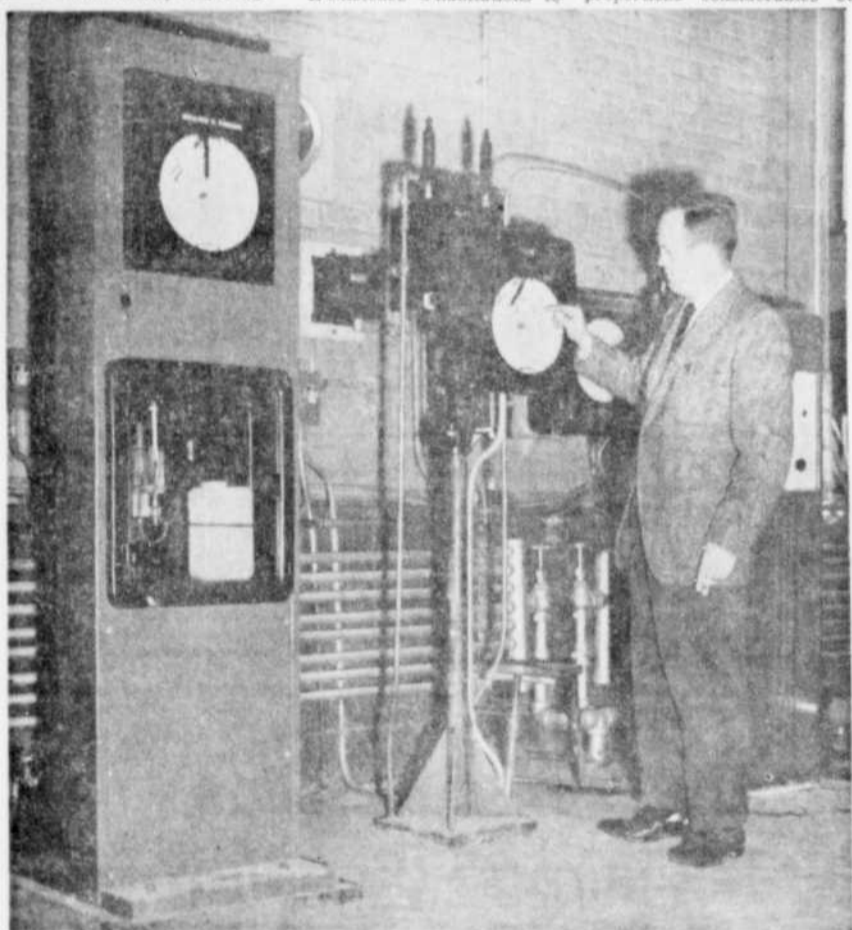
L'usine de pompage. — Cette photo a été prise à l'usine de pompage de Sherbrooke, construite en 1968. L'eau destinée à pourvoir aux besoins de la population subit un seul traitement, à savoir la chloration. On voit ici M. Jean-Paul Lajoie, ing. p., prenant connaissance de la consommation d'eau, soit alors neuf millions de gallons.
