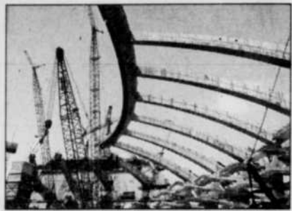
La structure du Stade olympique lors de sa construction.
