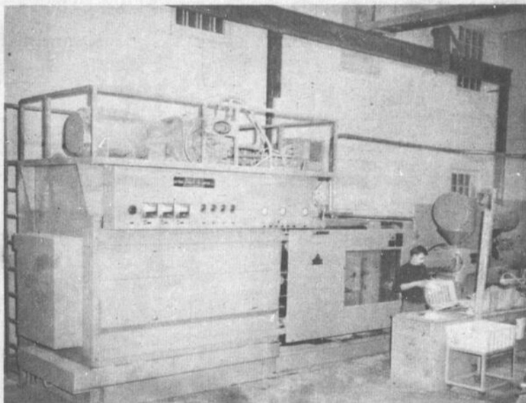
Machine à injection pour la fabrication d'objets de plastiques, telles caisses de liqueurs, chaudières ou chaises, comme celle que l'on vient de retirer de la machine.
