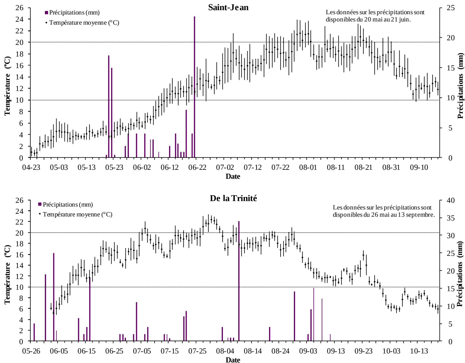
Figure 3. Précipitations et température journalière de l'eau des rivières Saint-Jean et de la Trinité en 2019
