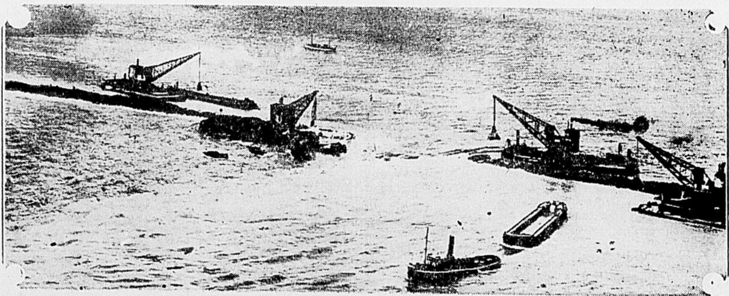
En Hollande, le peuple lutte continuellement contre l'invasion des eaux de la mer. On est en train de finir un barrage qui permettra l'établissement de milliers de fermes dans la partie desséchée.
