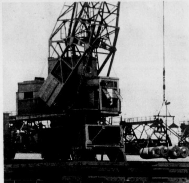
LA MÉTHODE NORMALE des chargements s'effectue par des grues pouvant manipuler de deux à quatre rouleaux de papier, alors que le nouveau système autorise une charge de douze.
