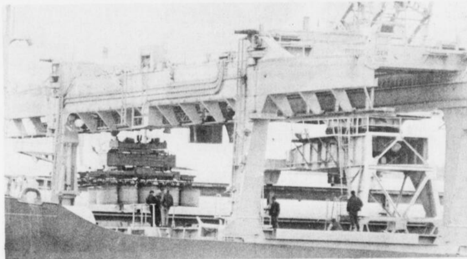
CETTE GRUE GÉANTE qui équipe les nouveaux navires de la "Star Shipping", souleve 12 rouleaux de papier journal à la fois. Elle est opérée par un employé seulement. Des ingénieurs et des spécialistes ont observé le comportement de l'appareil. On dit que la première expérience a donné d'heureux résultats.
