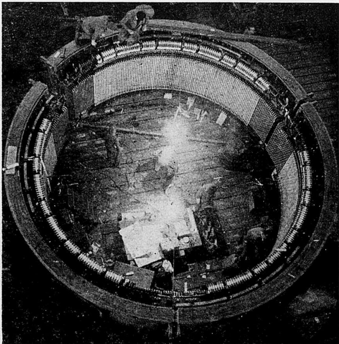
A l'usine Rade Koncar, un assemblage des milliers de fils d'un gros générateur d'énergie électrique.
