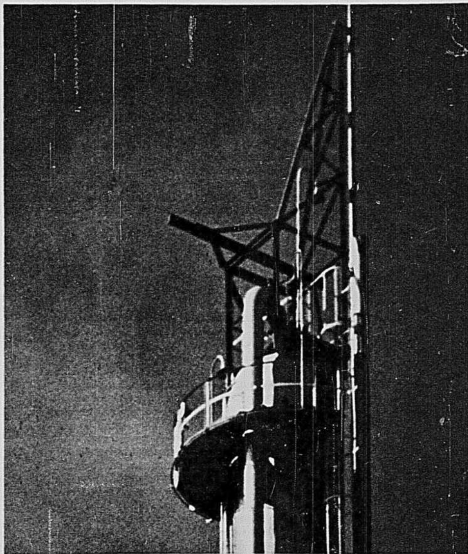
Cet alambic géant accomplit le dernier raffinage du pétrole; il en sort une gazoline à très haut indice d'octane. L'appareil de l'Imperial Oil a une capacité de 8,500 barils par jour.
