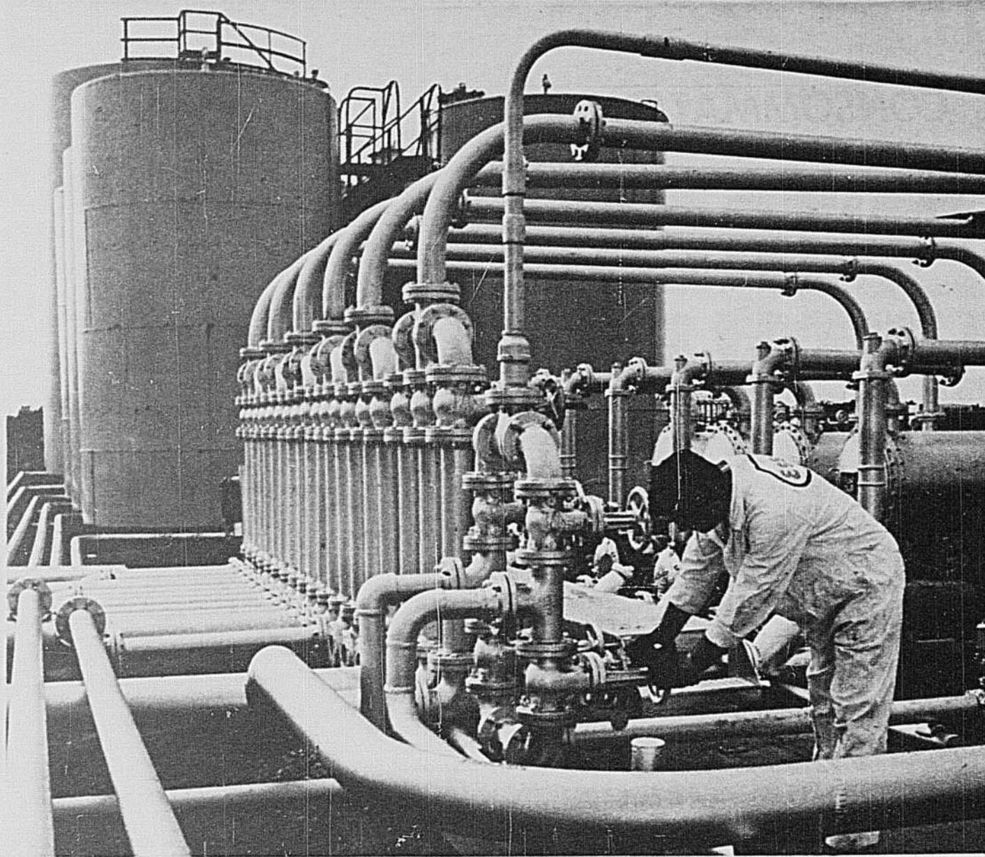
Les divers produits sortant de tel ou tel appareil de raffinage doivent être acheminés vers des réservoirs ou d'autres appareils qui les transformeront davantage. C'est un problème de circulation d'une incroyable complexité.
