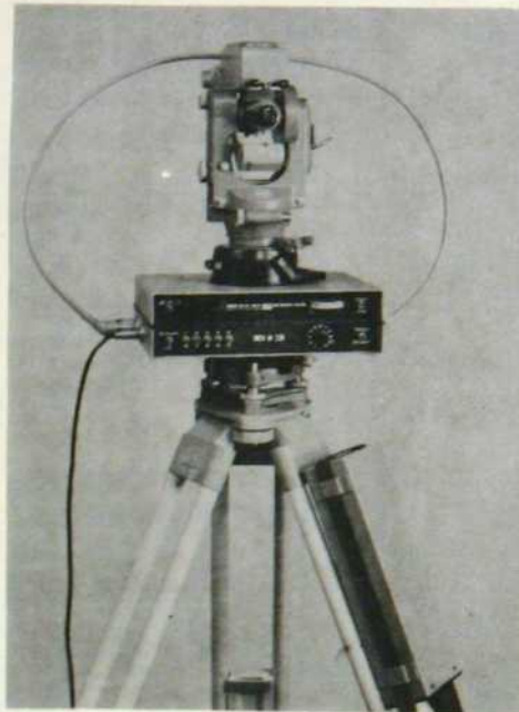
Dispositif de mesures à distance wild Di IOT sur théodolite Universel wild T2
