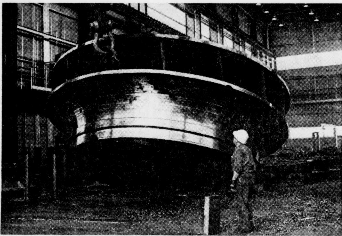
Cette roue de turbine en acier inoxydable et pesant 145 tonnes, coulée d'une seule pièce en 1969, a été installée à la centrale hydro-électrique de Churchill Falls.
