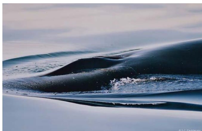
Photographie d'un rorqual commun prise par Stéphanie Pieddesaux lors d'une sortie en mer
