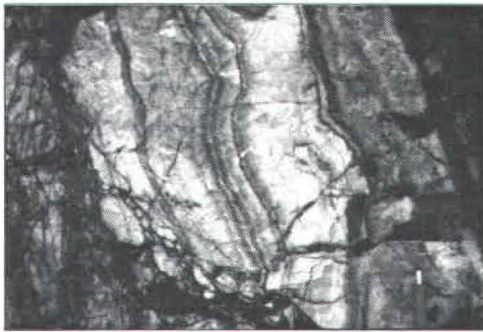
Veine de quartz-adulaire-hématite rubanée: exemple classique de minéralisation aurifère épithermale d'âge tardi-protérozoïque. Indice Steep Nap, zone d'Avalon, Terre-Neuve.
