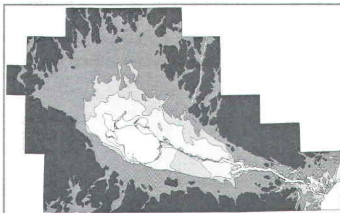
Carte d'analyse topographique mettant en relief l'effondrement du graben du Saguenay
