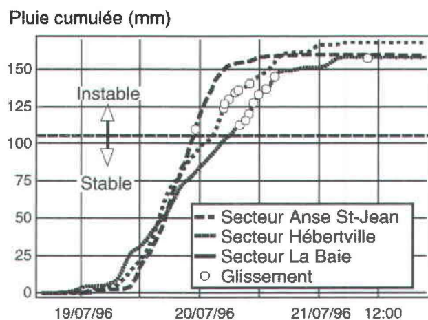
Relation entre la quantité de pluie tombée et le déclenchement des glissements de terrain. Le seuil de précipitation fixé à 100 mm ne s'applique qu'aux événements de la mi-juillet 1996.
