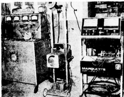
Machine infra-rouge pour la détection de dépense excessive et machine pour ajuster les lumières.
