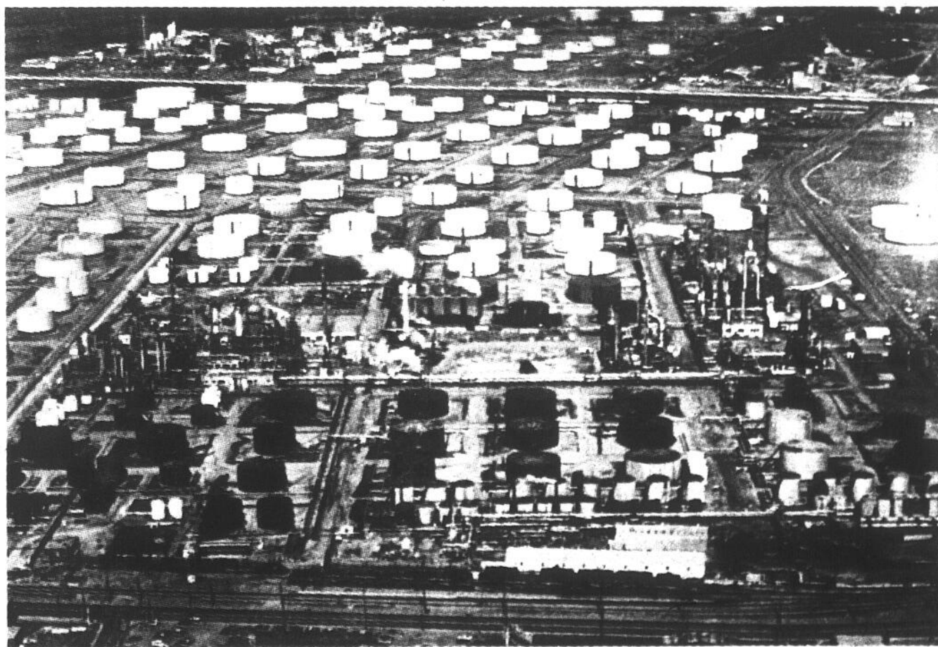
La raffinerie Gulf de Montréal-Est. Très impressionnante, cette vue aérienne ne montre toutefois, à peu près, que des réservoirs. Il en faut beaucoup pour une raffinerie comme celle-ci, qui produit environ 83,000 barils de produits pétroliers par jour, en plus d'entreposer du brut et des produits finis.
